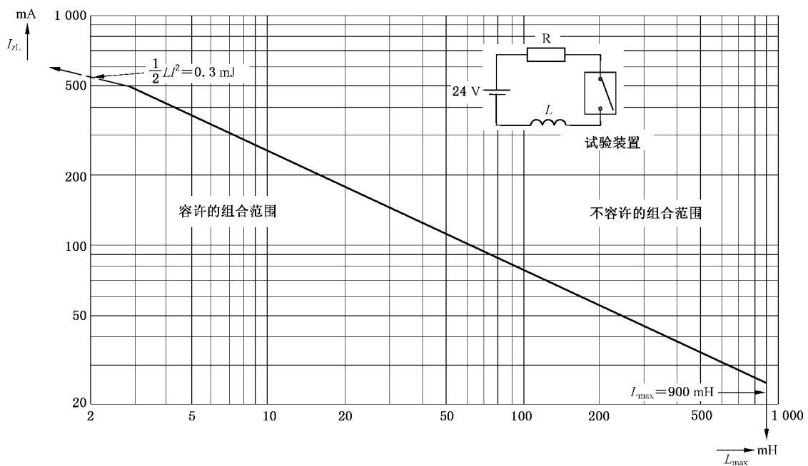
图 G.3 在乙醚蒸气和空气混合成的最易燃气体中电感电路上测得的最大容许电流 I_{zl} 和电感 L_{max} 的函数关系
