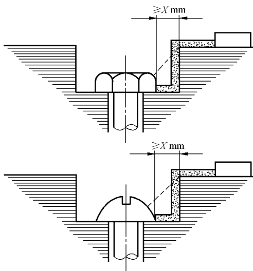
图 29 爬电距离和电气间隙——示例 8
