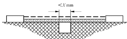
图 22 爬电距离和电气间隙——示例 1
