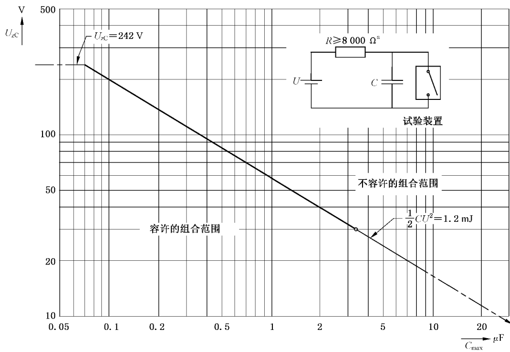
图 G.2 在乙醚蒸气和空气混合成的最易燃气体中电容电路上测得的最大容许电压 U_{xc} 和电容 C_{max} 的函数关系
