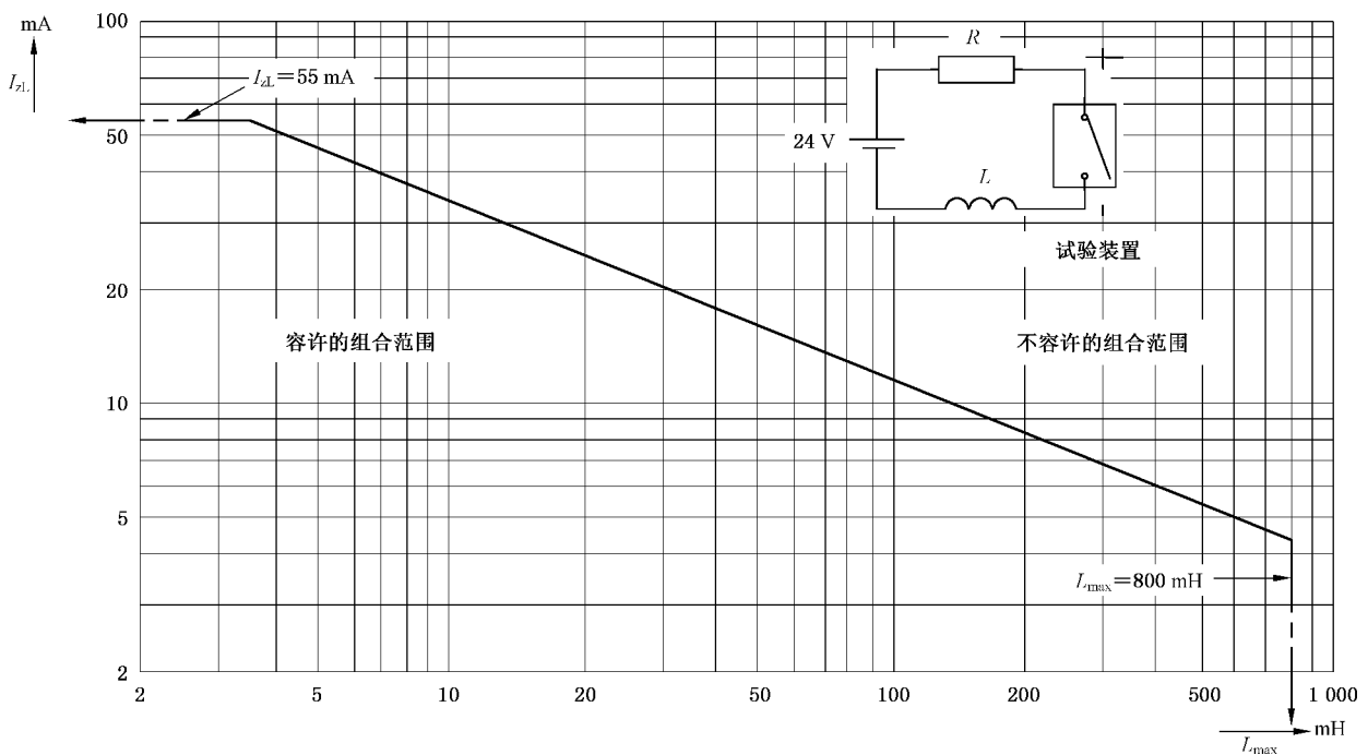
图 G.6 在乙醚蒸气和氧混合成的最易燃气体中电感电路上测得的最大容许电流 I_{zi} 和电感 L_{max} 的函数关系
